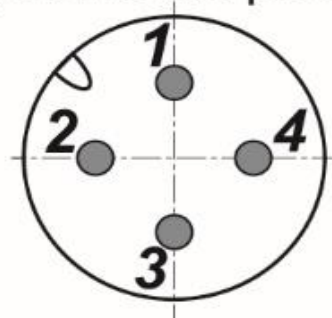
Цоколевка разъема
