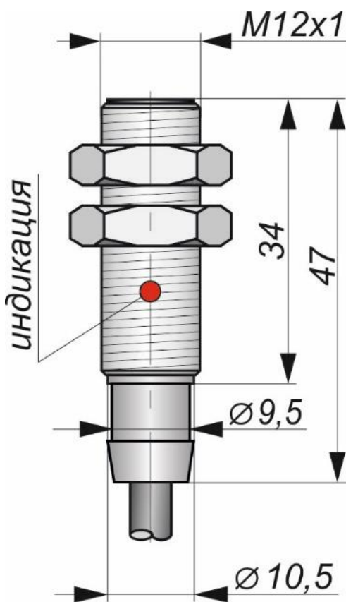
Габаритный чертеж
