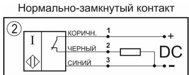
Схема соединения
