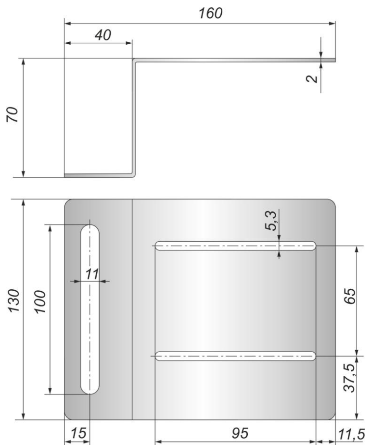
Габаритный чертеж
