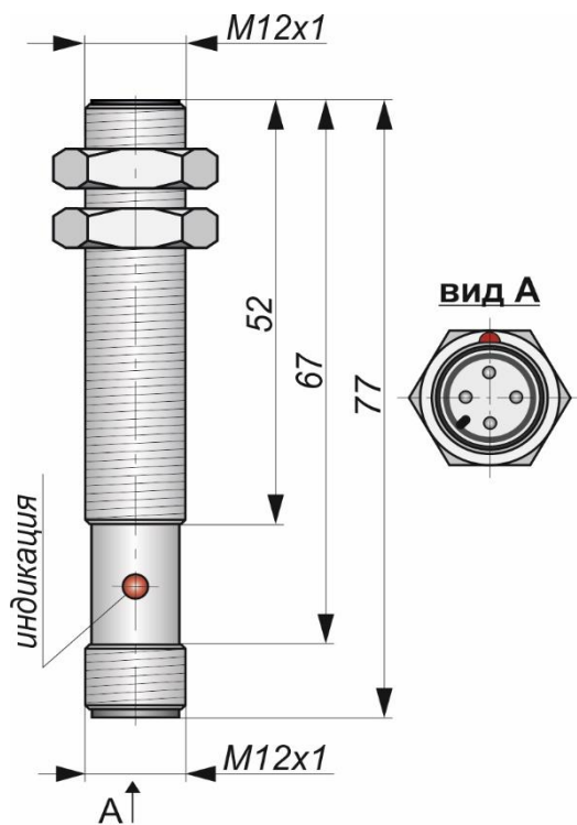
Габаритный чертеж
