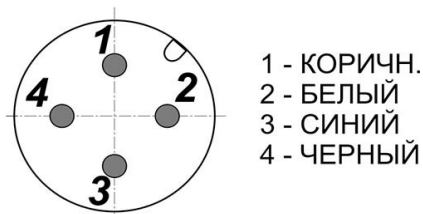
Цоколевка разъема
