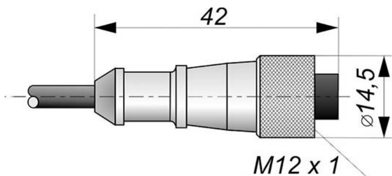
Габаритный чертеж
