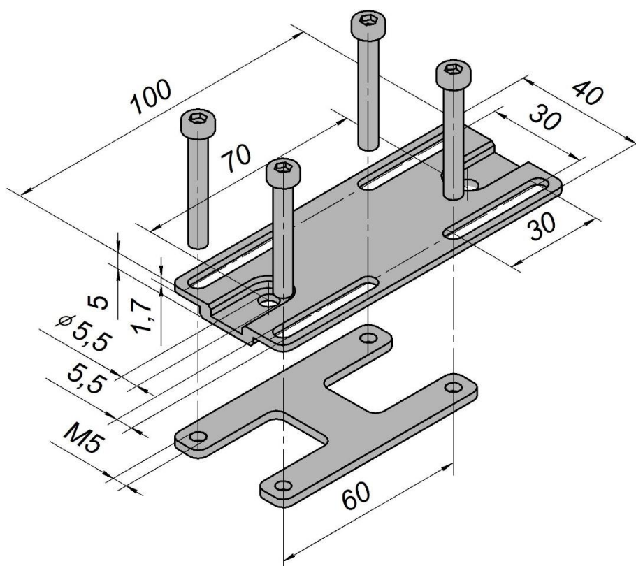
Габаритный чертеж
