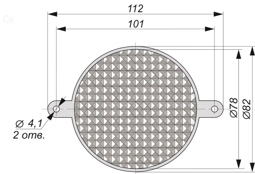
Габаритный чертеж
