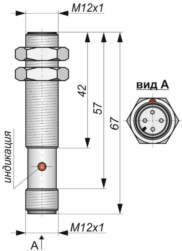
Габаритный чертеж
