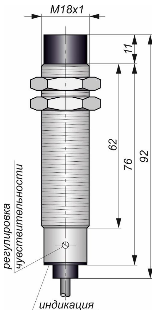
Габаритный чертеж
