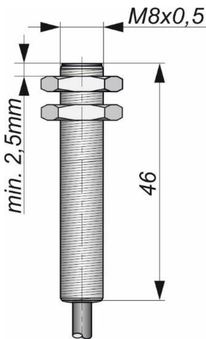
Габаритный чертеж
