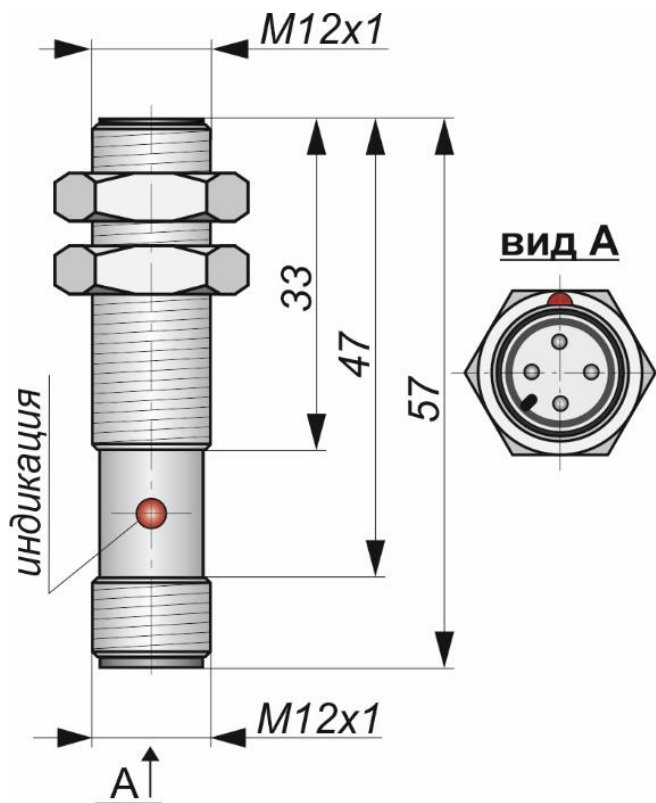
Габаритный чертеж
