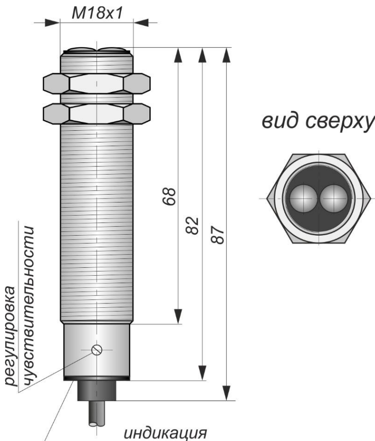
Габаритный чертеж
