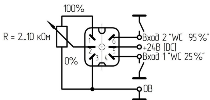
Схема подключения
