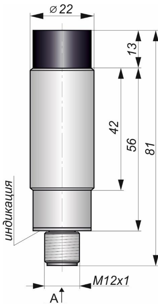
Габаритный чертеж
