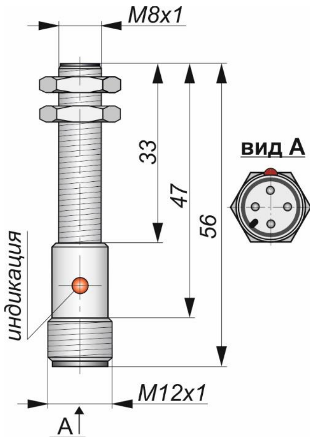
Габаритный чертеж
