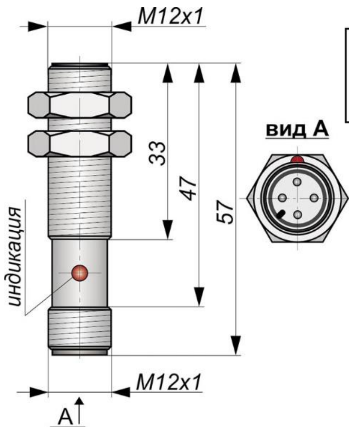
Габаритный чертеж
