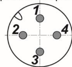
Цолевка разъема
