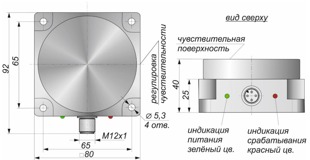
Габаритный чертеж
