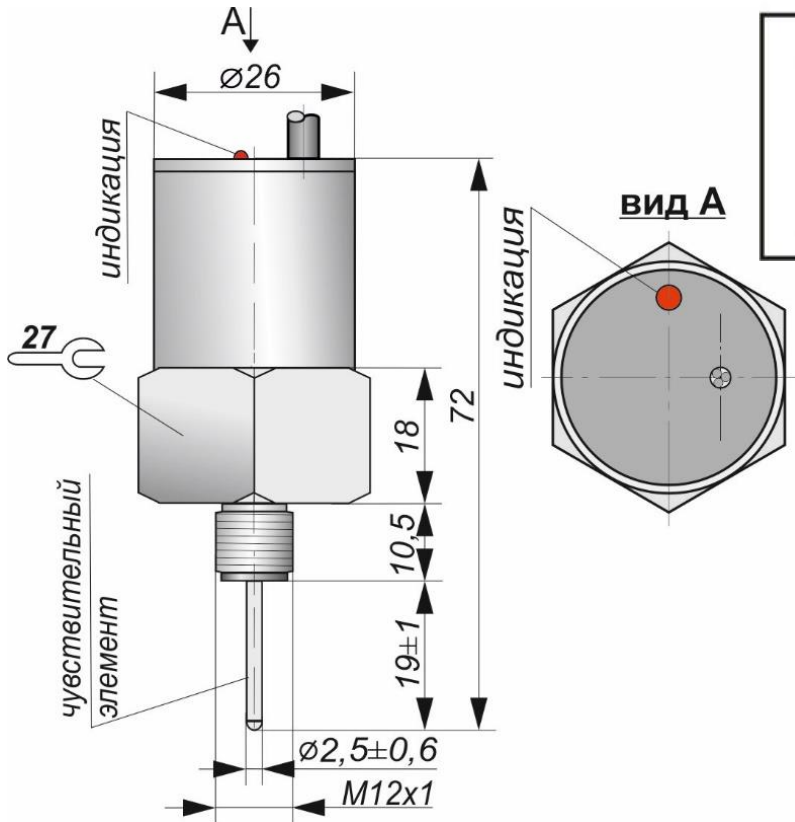
Габаритный чертеж
