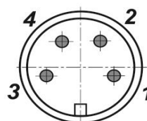
Цоколевка разъема
