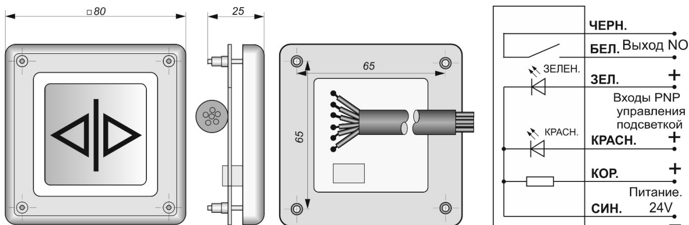
Габаритный чертеж
